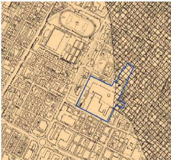
Carta microz.ne sismica livello 3°-Indice potenziale liquefazione Tav B
