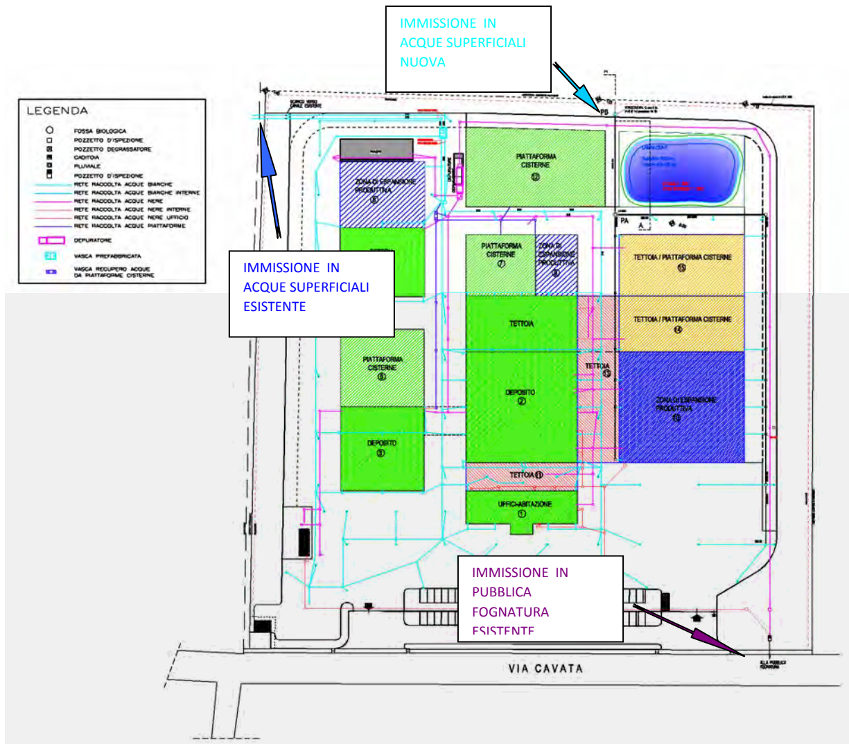
FIG. 3.24: PLANIMETRIA GENERALE RETI FOGNARIE ESISTENTI E DI PROGETTO
