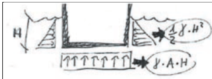
Figura 21: Schema concettuale delle forze agenti.
