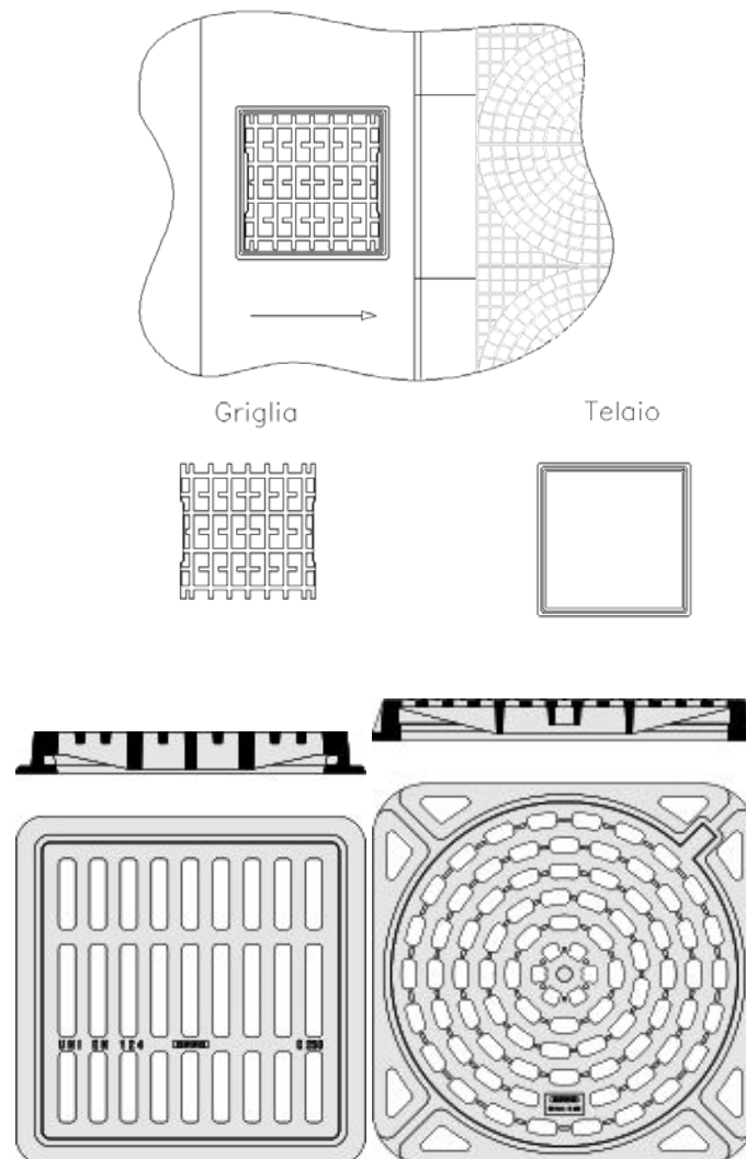
Figura 6: Tipologie di griglie di possibile adozione UNI EN 124 (waterway >700cmq).
