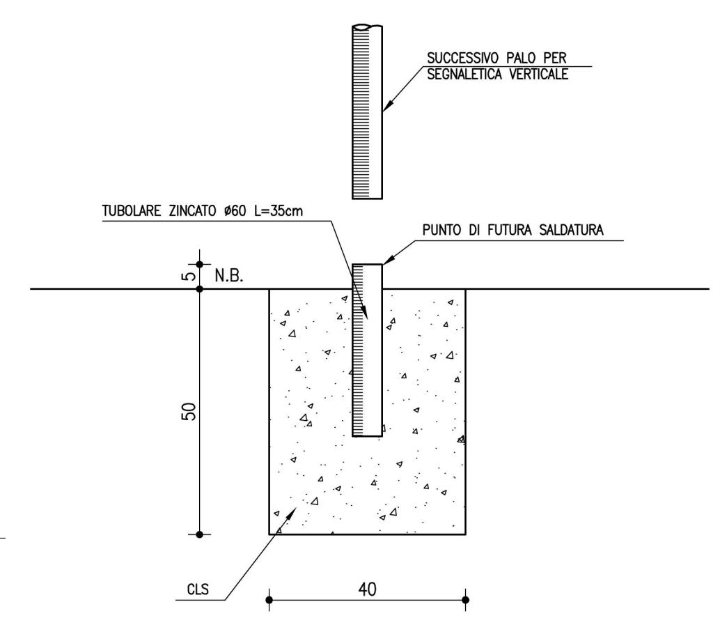
PLINTINI PER SEGNALETICA sezione trasversale 1:10
