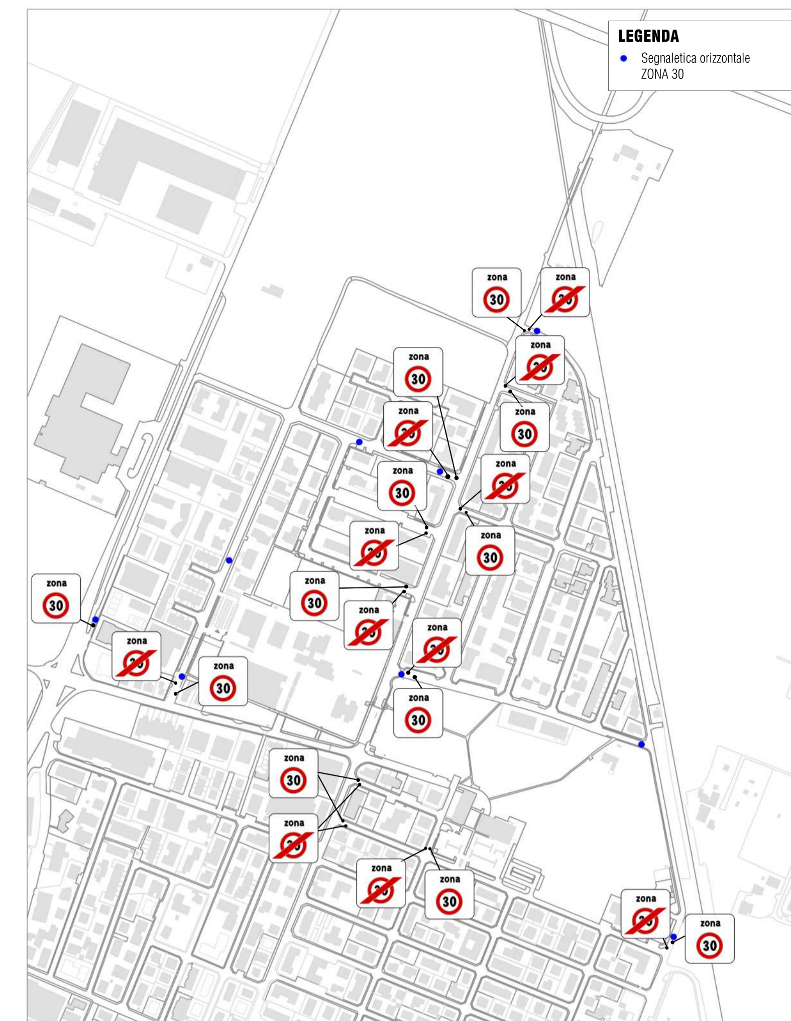
Planimetria generale - 1:5000
