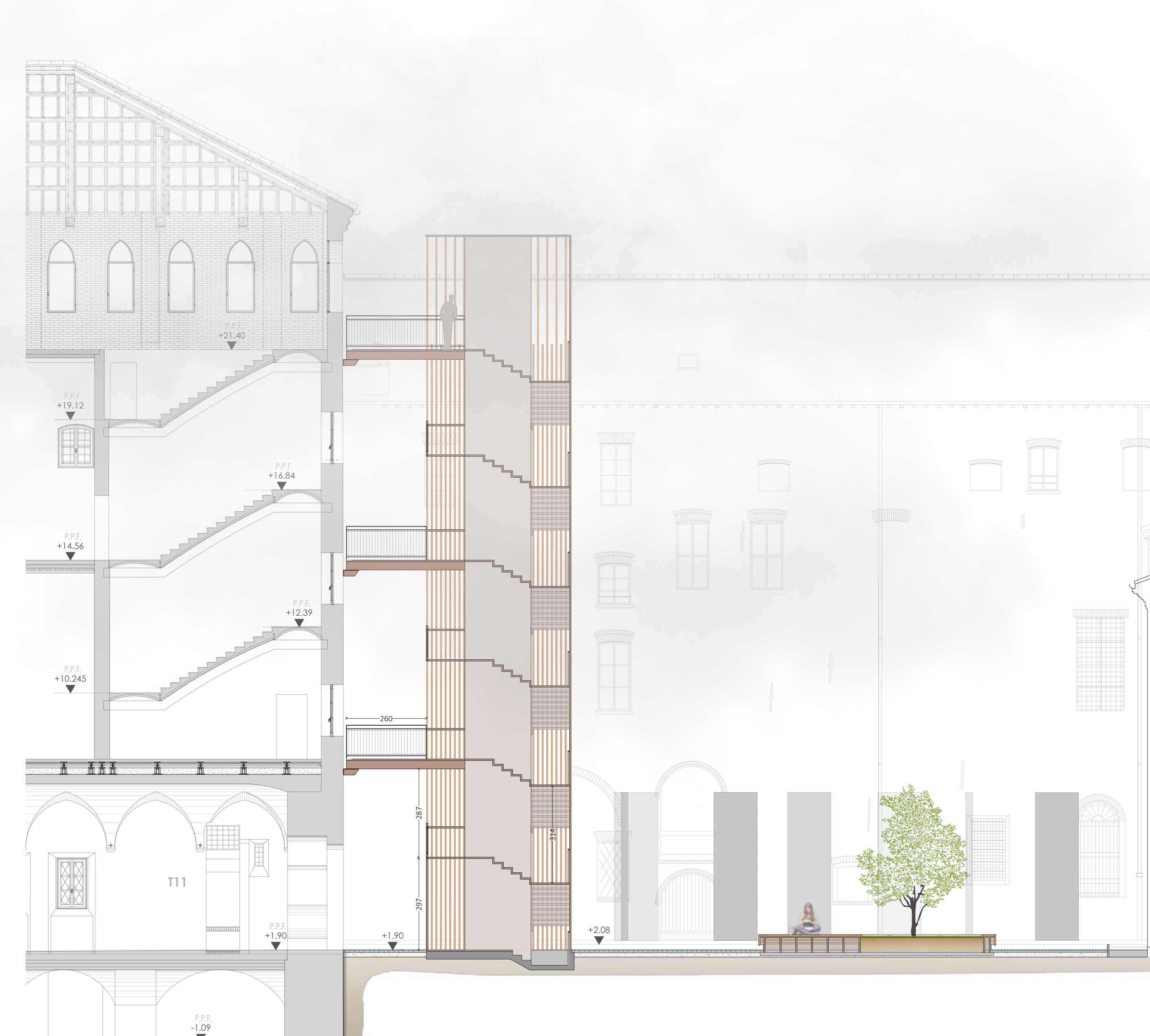
Sezione BB - area cortiliva
